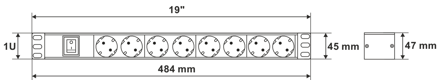
plug: type: E/F („Unischuko”)
